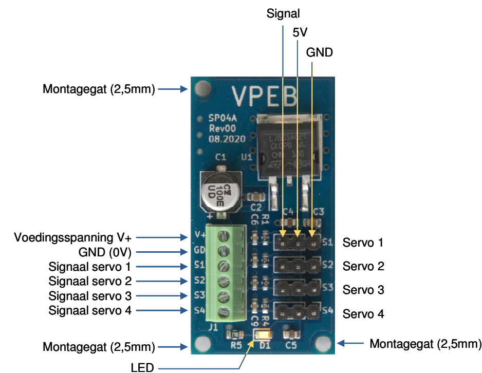
Afbeelding 2: SP04A overzicht aansluitingen en functies
