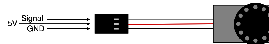
Afbeelding 3: Aansluitingen servo
